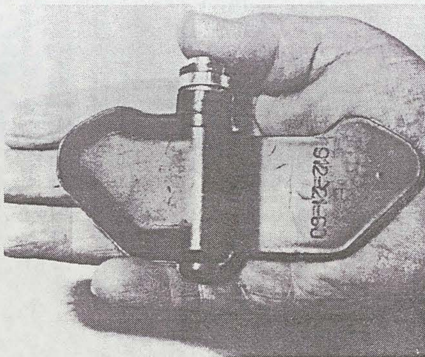
Figuur 6. De PFM-1S antipersoneelmijn (Dienstgeheim)
