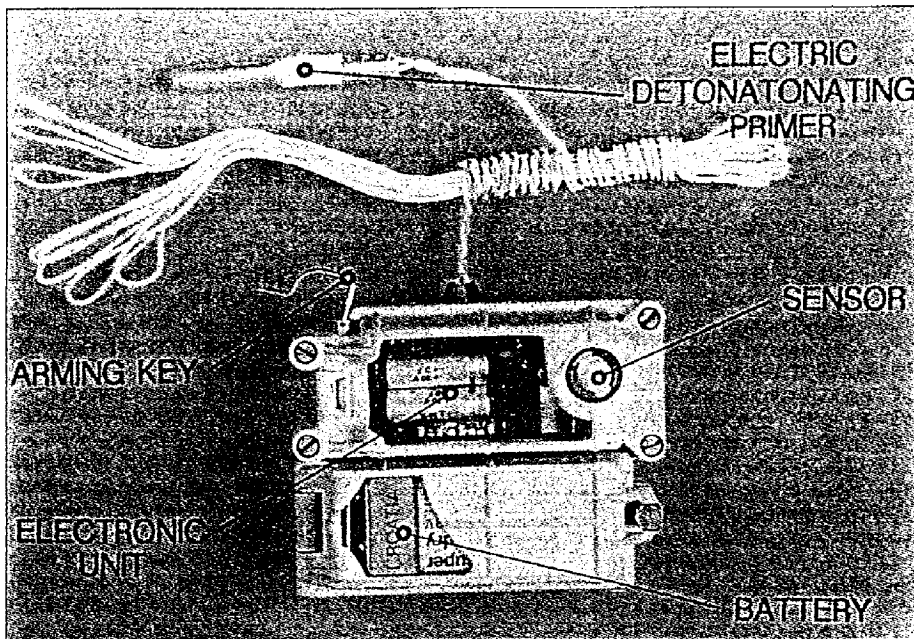
Op de foto zijn de verschillende delen van de USS-T elektronische ontsteker te zien. Het elektrische slagpijpje is aangesloten.
