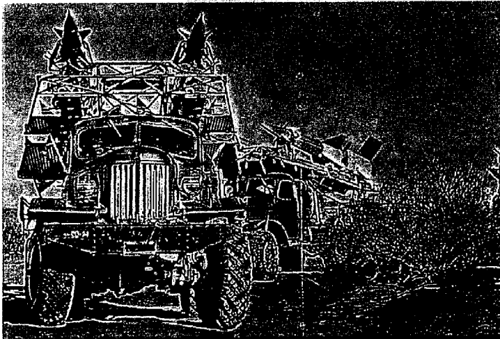
HERBEVOORRADINGSVOERTUIG ZIL-157
