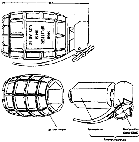
4 Tekening explosief.
